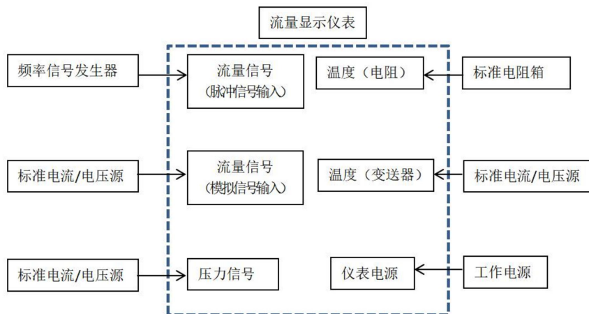
图 1 流量显示仪表校准接线示意图
